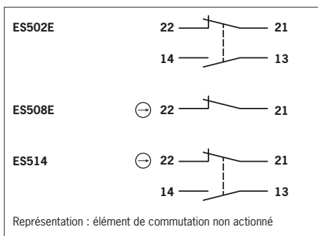
Fig. 1 : Éléments de commutation et affectation des broches
